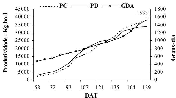
Figura 53 – Graus-dia e produtividade acumulada da cultura de pimentão em função do número de dias após o transplante, nos dois sistemas de plantio.
