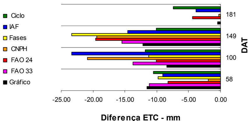
Figura 47 - Comparação entre os métodos de determinação do Kc, com relação à subestimativa da ETC por ciclo de produção, no sistema de plantio convencional.
