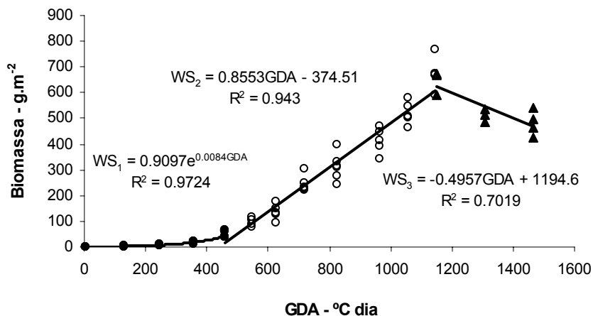
Figura 55 - Modelos ajustados para descrever biomassa acumulada pela planta em função de graus-dia acumulados.
