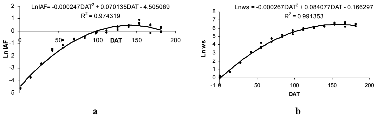
Figura 23 – Modelos de ajuste de IAF (a) e biomassa (b) em função do tempo para o sistema de plantio direto.
