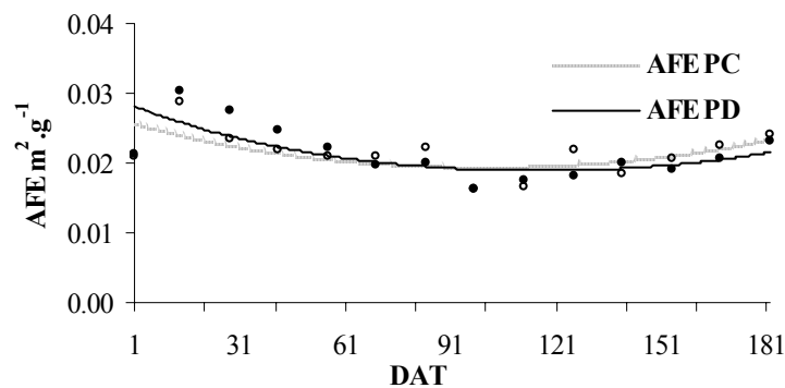
Figura 31 - Curvas de área foliar específica e seus valores médios observados na cultura do pimentão nos sistemas de plantio convencional (AFE PC) e direto (AFE PD).
