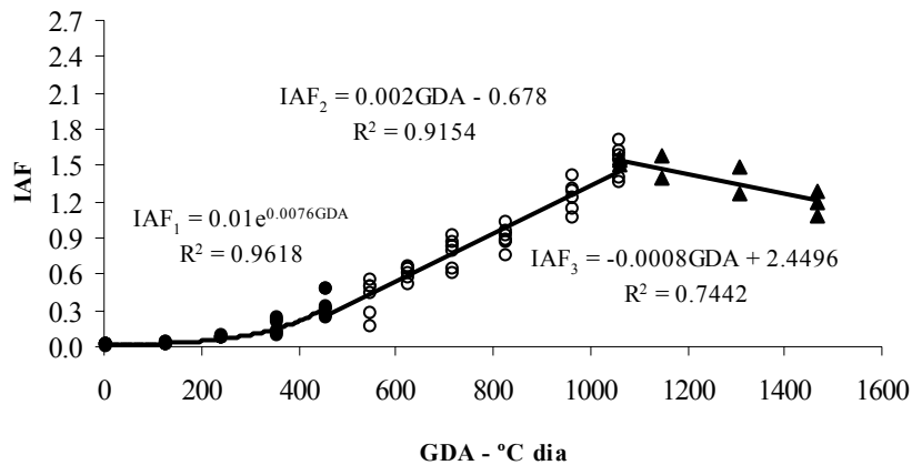
Figura 54 - Modelos ajustados para descrever IAF da cultura do pimentão em função de graus-dia acumulados.
