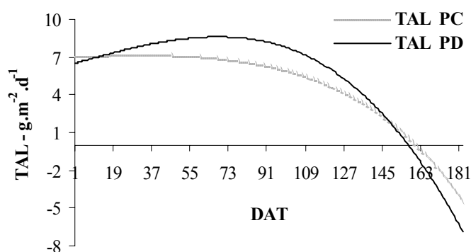
Figura 28 – Taxa de assimilação líquida da cultura em função de DAT.
