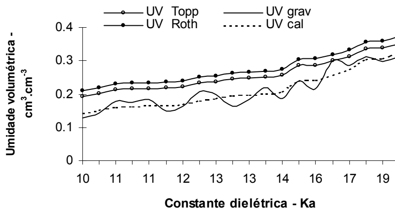
Figura 38 - Comparação dos modelos ajustados pela metodologia TDR em relação ao método gravimétrico, para a profundidade de 0,10m.
