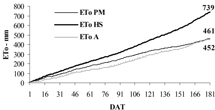
Figura 36 – Evapotranspiração de referência acumulada durante o ciclo da cultura do pimentão estimada pelos métodos Penman-Monteith (ETo PM), Hargreaves-Samani (ETo HS) e Tanque Classe “A” (ETo A).
