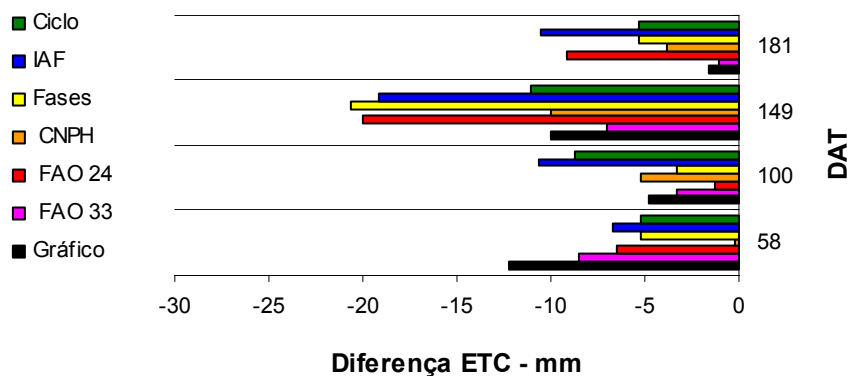
Figura 50 - Comparação entre os métodos de determinação do Kc, com relação à subestimativa da ETC por ciclo de produção, no sistema de plantio direto.
