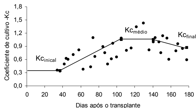
Figura 44 – Curva de Kc para a cultura do pimentão, no sistema de plantio direto.
