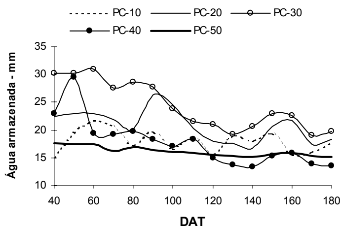
Figura 12 - Variação da lâmina armazenada no perfil do solo no sistema de plantio convencional nas profundidades de 0,10 a 0,50m (PC10 a PC50) utilizando TDR .
