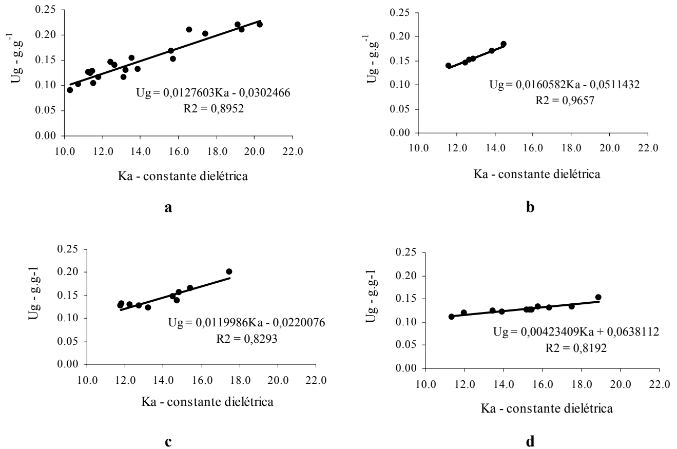
Figura 37 - Modelos de calibração para TDR para as profundidades de 0 a 0,20m (a), 0,20 a 0,30m (b), 0,30 a 0,40m (c) e 0,40 a 0,50m (d).
