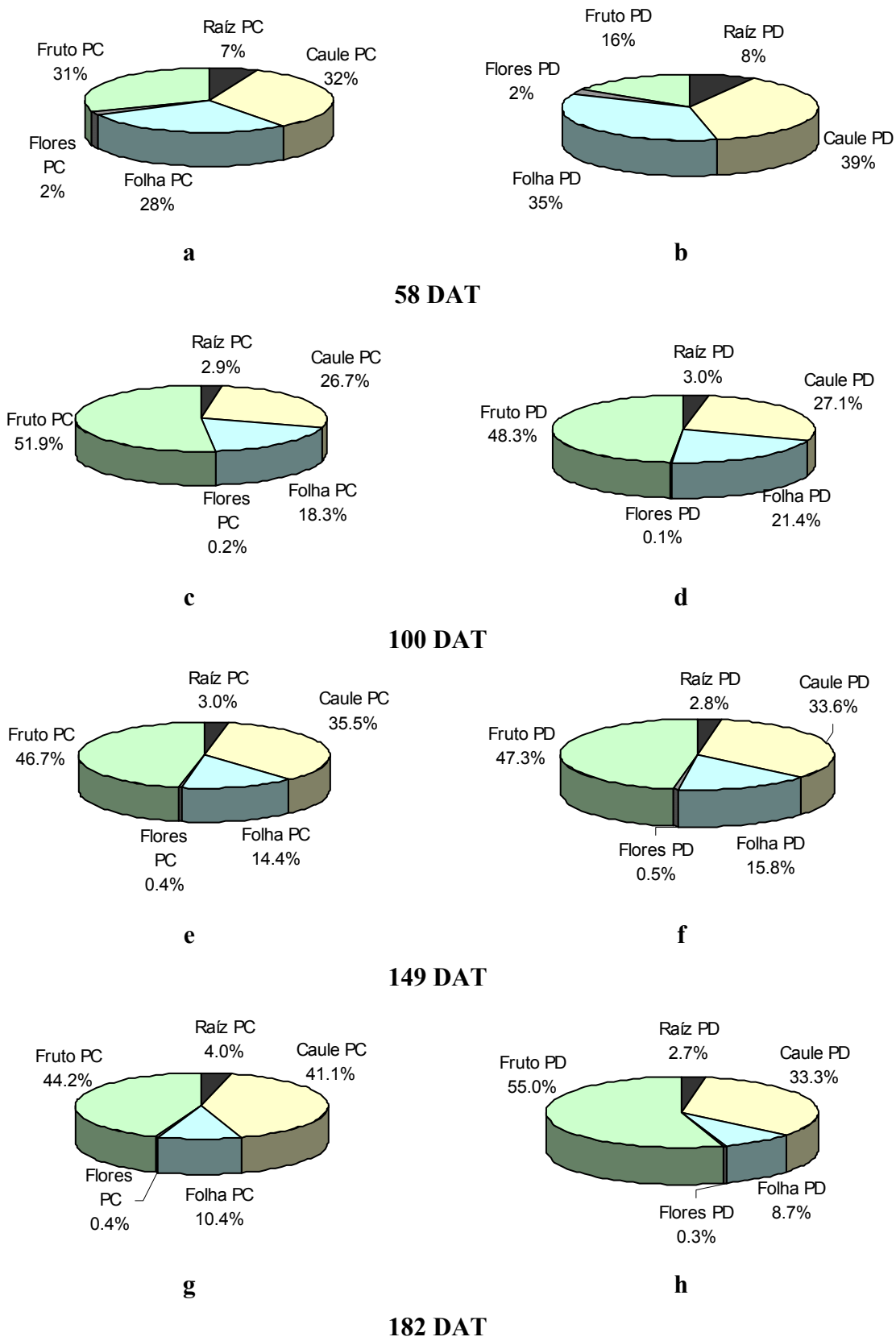
Figura 35 – Biomassa acumulada pelas partes da planta nos sistemas de plantio convencional (a, c, e, g) e direto (b, d, f, h), em diferentes fases de desenvolvimento da cultura do pimentão.
