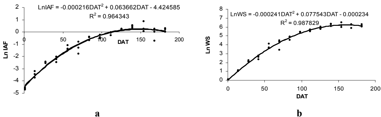
Figura 22 – Modelos de ajuste de IAF (a) e biomassa (b) em função do tempo para os sistema de plantio convencional.
