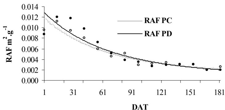
Figura 30 – Curvas de razão de área foliar e seus valores médios para a cultura do pimentão nos sistemas de plantio convencional (RAF PC) e direto (RAF PD).
