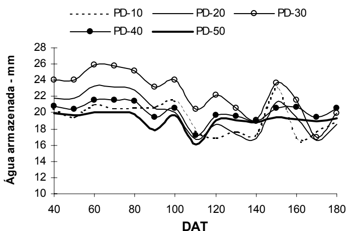
Figura 13 - Variação da lâmina armazenada no perfil do solo no sistema de plantio direto nas profundidades de 0,10 a 0,50m (PD10 a PD50) utilizando TDR.
