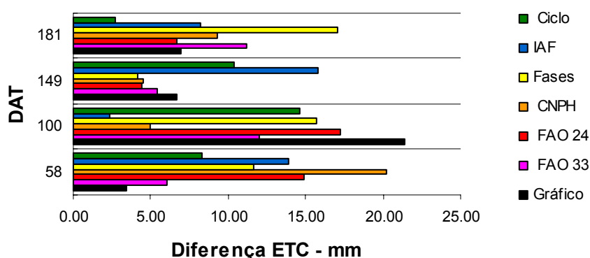
Figura 46 - Comparação entre os métodos de determinação do Kc, com relação à superestimativa da ETC por ciclo de produção, no sistema de plantio convencional.
