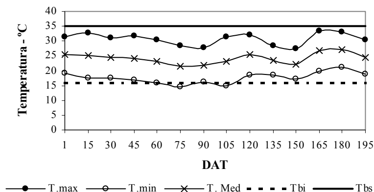
Figura 14 - Temperaturas Mínimas (Tmin), máximas (Tmax), médias (Tmed), e basal inferior (Tbi) e basal superior (Tbs) durante o ciclo da cultura do pimentão no sistema de plantio convencional e direto.
