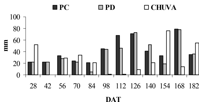
Figura 39 - Precipitação pluviométrica e lâminas de irrigação aplicadas nas parcelas sob sistema de plantio convencional (PC) e direto (PD).
