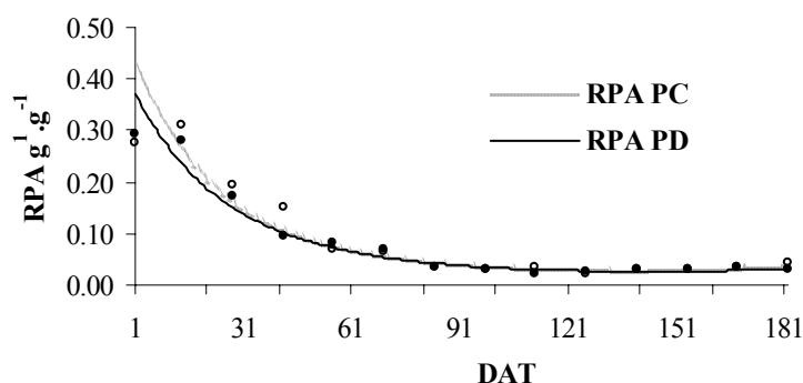
Figura 33 - Relação Raiz Parte Aérea da cultura do pimentão nos sistemas de plantio convencional (RPA PC) e direto (RPA PD). Os círculos são as médias observadas no plantio convencional e os pontos no plantio direto.
