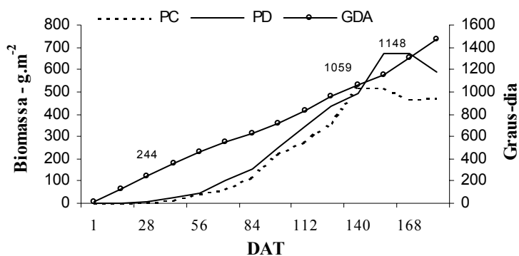
Figura 51 – Graus-dia e biomassa acumulada pela cultura do pimentão em função de dias após o transplante.
