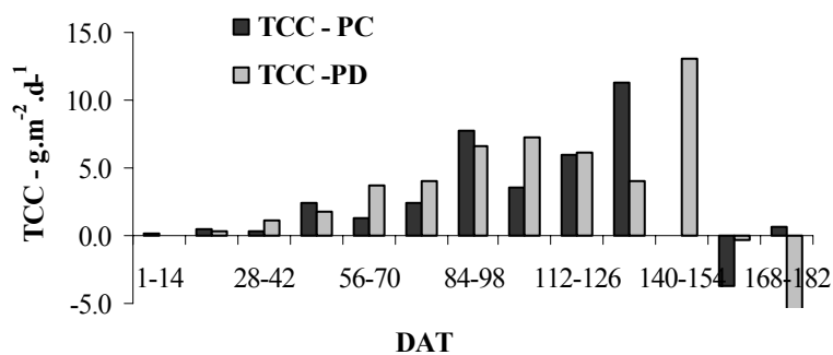
Figura 19 - Taxa de crescimento da cultura do pimentão nos sistemas de plantio convencional (TCC-PC) e direto (TCC-PD).
