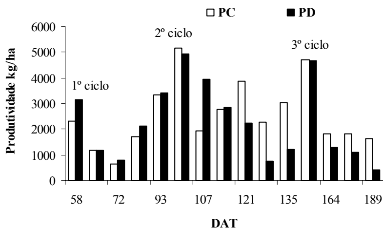
Figura 34 – Produtividade da cultura do pimentão nos sistemas de plantio convencional (PC) e direto (PD).
