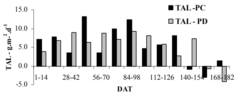
Figura 20 - Taxa de assimilação líquida da cultura do pimentão nos sistemas de plantio convencional (TAL-PC) e direto (TAL-PD)
