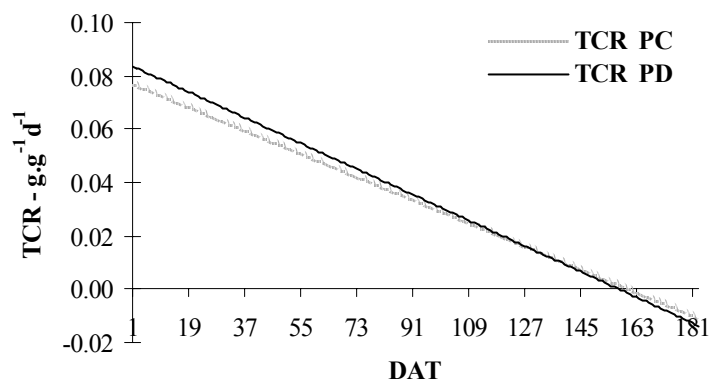
Figura 27 – Taxa de crescimento relativo da cultura em função de DAT.
