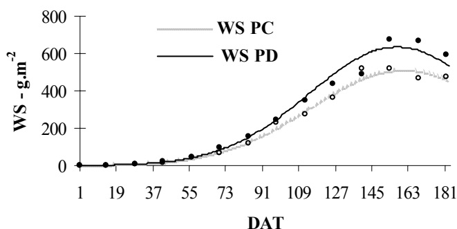
Figura 24 – Valores médios observados e ajustados de biomassa (WS) acumulada em função de DAT, para o plantio direto (PD) e convencional (PC).
