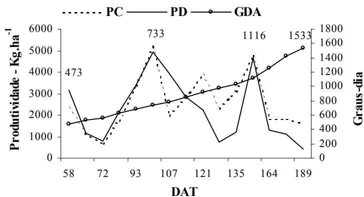
Figura 52 – Graus-dia e colheitas de pimentão em função de dias após o transplante nos dois sistemas de plantio.
