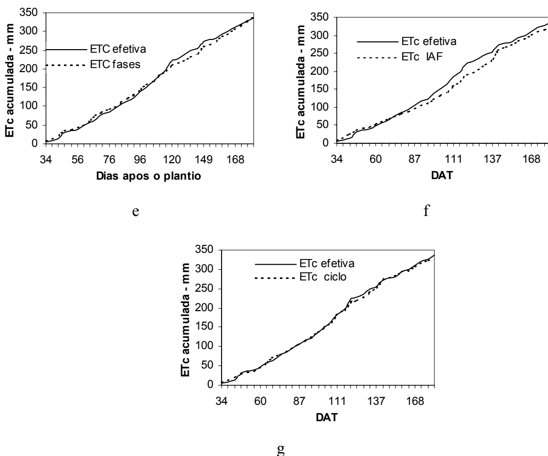
Figura 45 - Comparação da ETc efetiva acumulada com as ETc's calculadas e acumuladas pelas metodologias do Gráfico (a), FAO 33 (b), FAO 24 (c), CNPH (d), Fases (e), IAF (f) e Ciclo (g), no sistema de plantio convencional.
