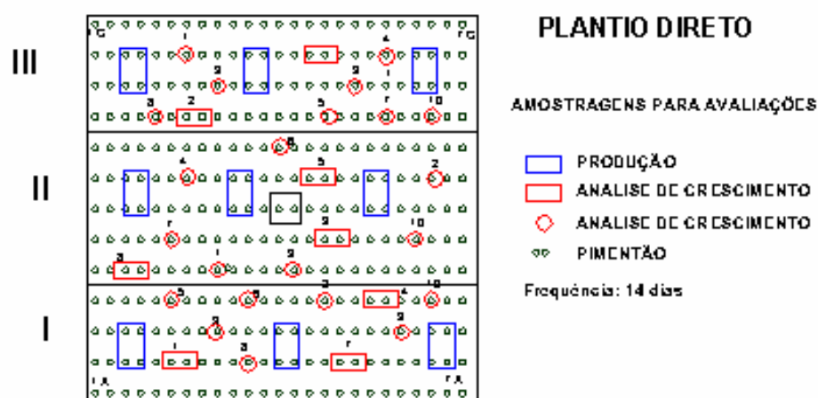
Figura 16 – Esquema de coletas para análise de crescimento e disposição das plantas nas repetições I, II e III, no sistema de plantio direto.
