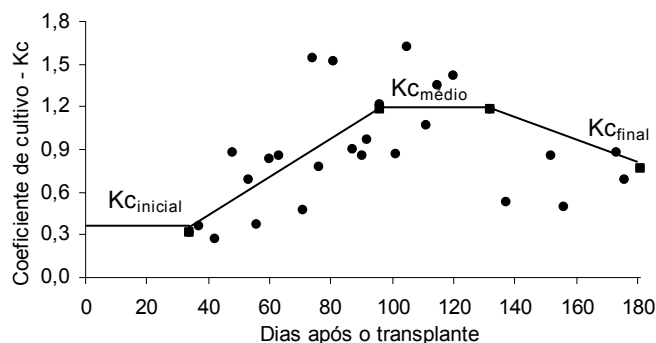
Figura 43 – Curva de Kc para a cultura do pimentão, no sistema de plantio convencional.
