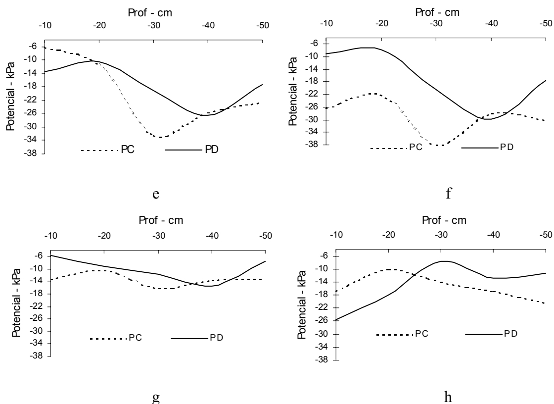
Figura 40 – Variação de potencial matricial no PC e PD da água no perfil do solo, aos 28(a), 70(b), 84(c), 98(d), 126(e), 140(f), 168(g) e 182(h) DAT.
