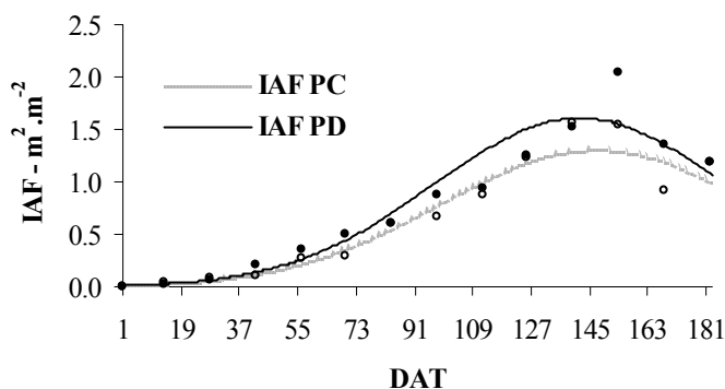
Figura 25 – Valores médios observados e ajustados de índice de área foliar em função de DAT, para o plantio direto (PD) e convencional (PC).
