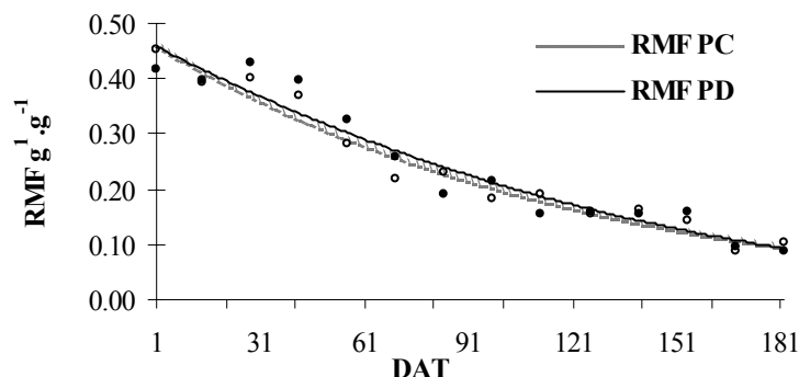
Figura 32 - Razão de massa foliar da cultura do pimentão nos sistemas de plantio convencional (RMF PC) e direto (RMF PD). Os círculos são as médias observadas no plantio convencional e os pontos no plantio direto.
