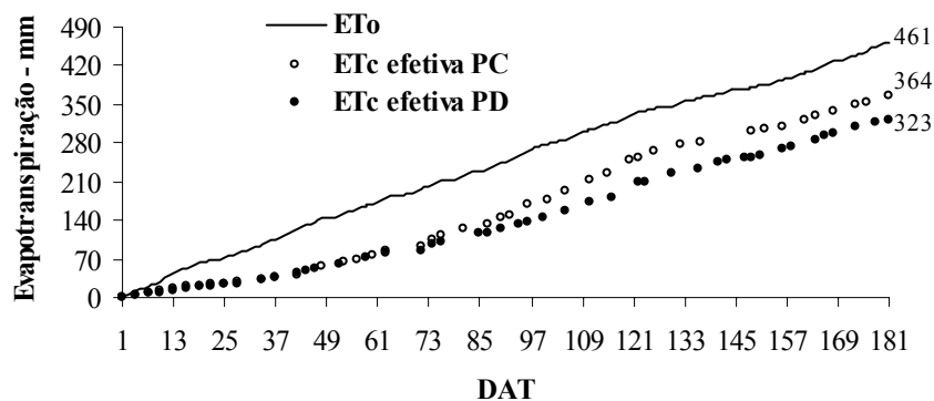
Figura 42 – Valores acumulados de evapotranspiração de referência e evapotranspiração efetiva da cultura do pimentão, no sistema de plantio convencional e direto, durante a execução do experimento.
