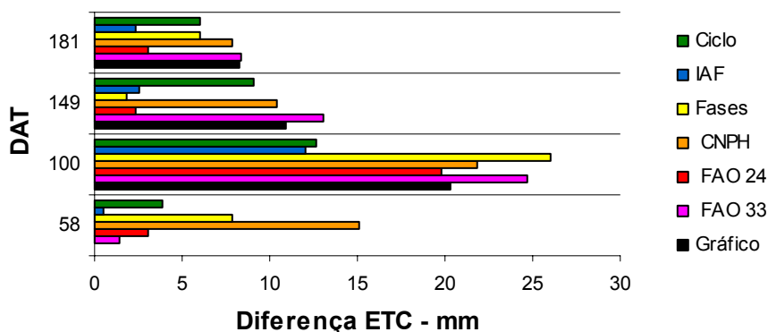
Figura 49 - Comparação entre os métodos de determinação do Kc, com relação à superestimativa da ETC por ciclo de produção, no sistema de plantio direto.
