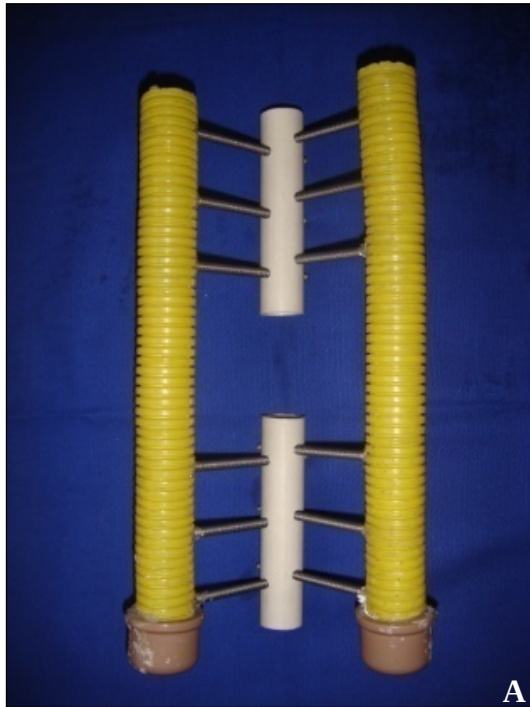
Figura 13 – A) Foto de corpo de prova de aparelho de fixação esquelética externa com barra de conexão de resina acrílica autopolimerizável e 12 pinos de inserção (seis por fragmento/ três por barra estabilizadora em cada fragmento). B) Esquema de montagem do mesmo aparelho. Valores expressos em centímetros.
