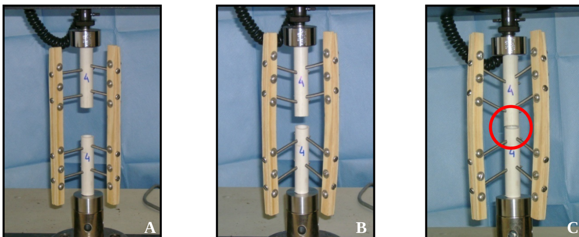
Figura 20 – Seqüência do teste de compressão axial do corpo de prova número quatro pertencente ao grupo A (corpos de prova com aparelhos de fixação esquelética externa confeccionados com barras de conexão de madeira e oito pinos de inserção - quatro por fragmento/ dois por barra estabilizadora em cada fragmento). A) Início do teste, B) Angulação dos pinos de inserção, C) Contato dos fragmentos, determinando o término do ensaio.
