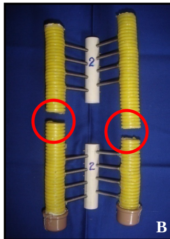
Figura 26 – Seqüência do teste de compressão axial do corpo de prova número dois pertencente ao grupo F (corpos de prova com aparelhos de fixação esquelética externa confeccionados com barras de conexão de resina acrílica autopolimerizável e 16 pinos de inserção - oito por fragmento/ quatro por barra estabilizadora em cada fragmento). A) Início do teste, B) Após o término do ensaio, caracterizado pela falha do aparelho.
