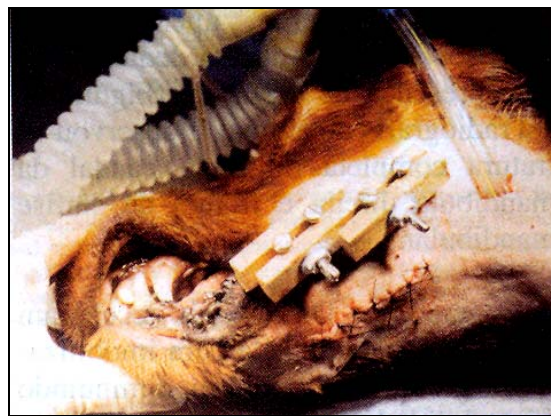
Figura 3 – Aparelho de fixação esquelética externa confeccionado com barras de conexão de madeira ( Pinnus ellioti ) utilizado para fixação de fraturas mandibulares em cão. Fonte: Botelho et al. (2001).
