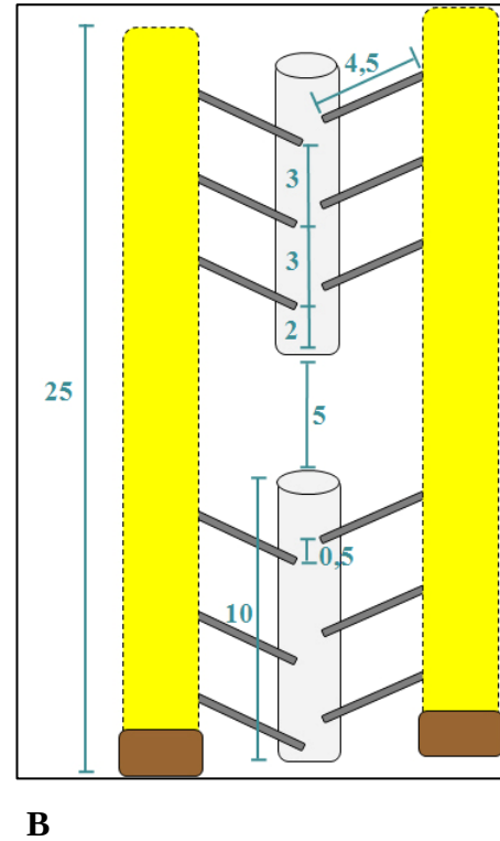
Figura 13 – A) Foto de corpo de prova de aparelho de fixação esquelética externa com barra de conexão de resina acrílica autopolimerizável e 12 pinos de inserção (seis por fragmento/ três por barra estabilizadora em cada fragmento). B) Esquema de montagem do mesmo aparelho. Valores expressos em centímetros.
