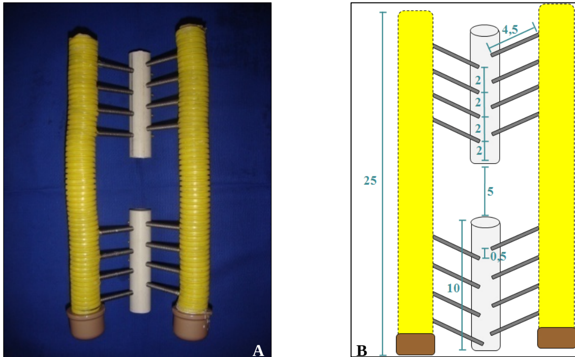
Figura 14 – A) Foto de corpo de prova de aparelho de fixação esquelética externa com barra de conexão de resina acrílica autopolimerizável e 16 pinos de inserção (oito por fragmento/ quatro por barra de conexão em cada fragmento). B) Esquema de montagem do mesmo aparelho. Valores expressos em centímetros.
