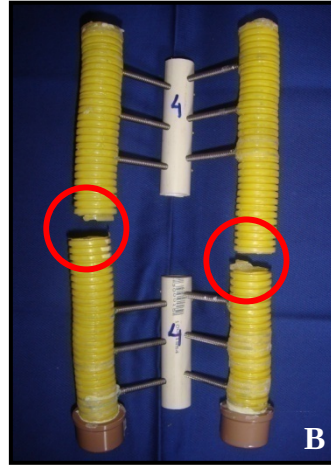
Figura 25 – Seqüência do teste de compressão axial do corpo de prova número quatro pertencente ao grupo E (corpos de prova com aparelhos de fixação esquelética externa confeccionados com barras de conexão de resina acrílica autopolimerizável e 12 pinos de inserção - seis por fragmento/ três por barra estabilizadora em cada fragmento). A) Início do teste, B) Após o término do ensaio, caracterizado pela falha do aparelho.
